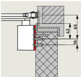
Beispiel: DIN-L-Tür, DIN-R-Tür spiegelbildlich
